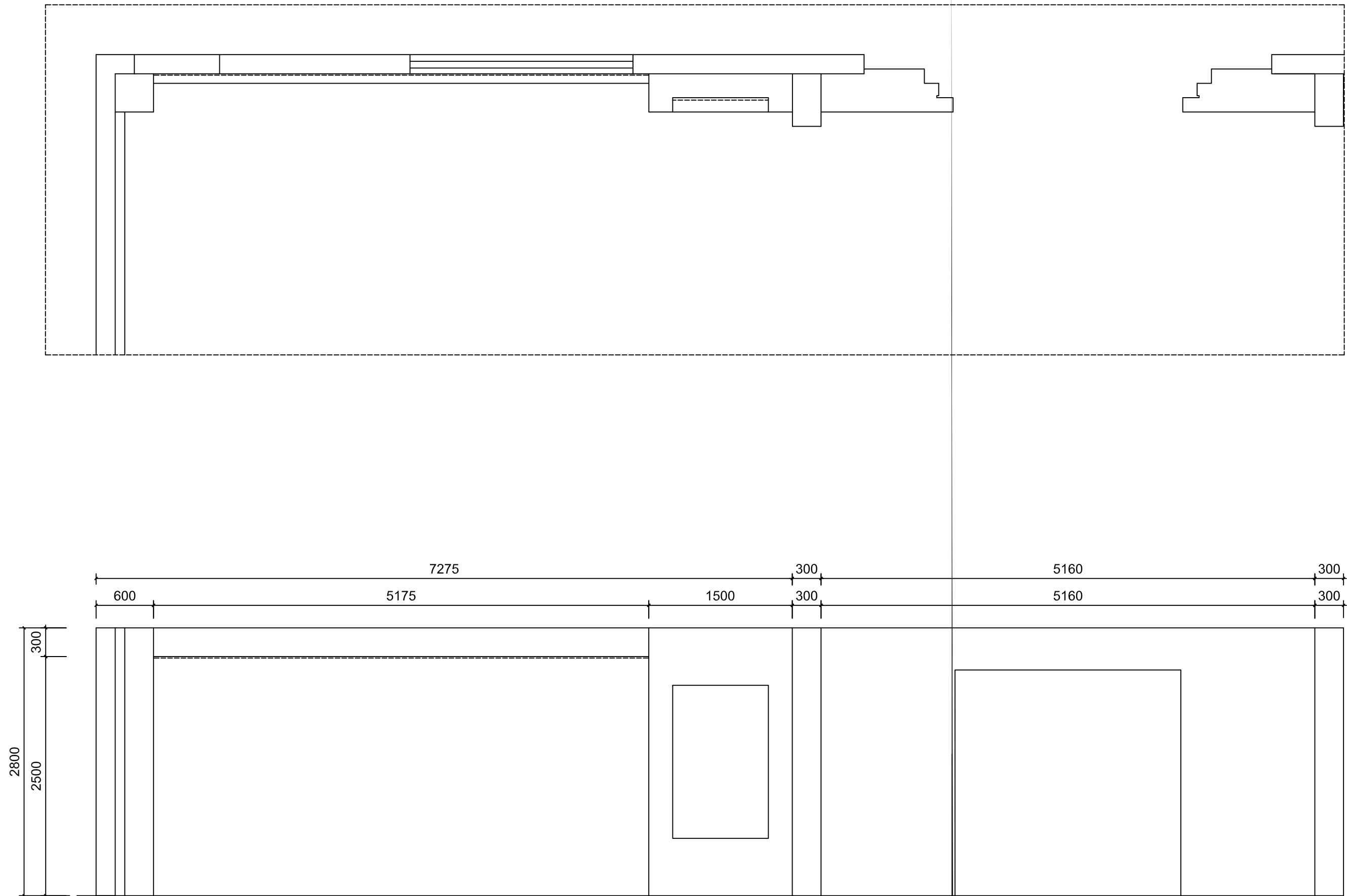
立面图A13
